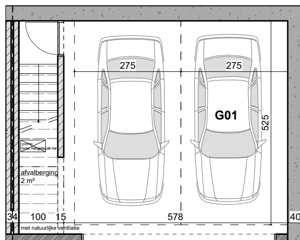
grondplan garage -01
